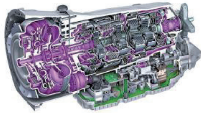
Resim 2: Sadece bir yağ ile şanzıman yıkama işlemi sırasında şanzımanın içi de (mor alan) temizlenir
